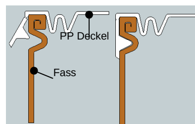
Geöffneter/geschlossener Deckel
